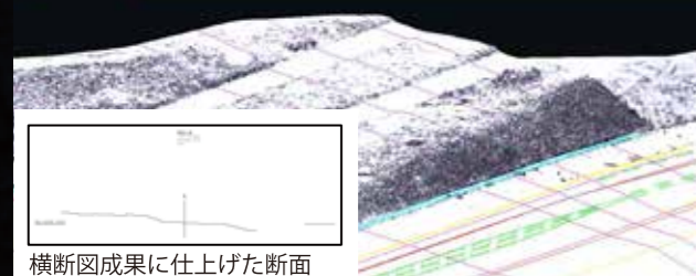
線形路線に沿って登録された横断線
