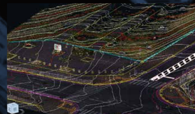
間引きを行った点群から作成した等高線
