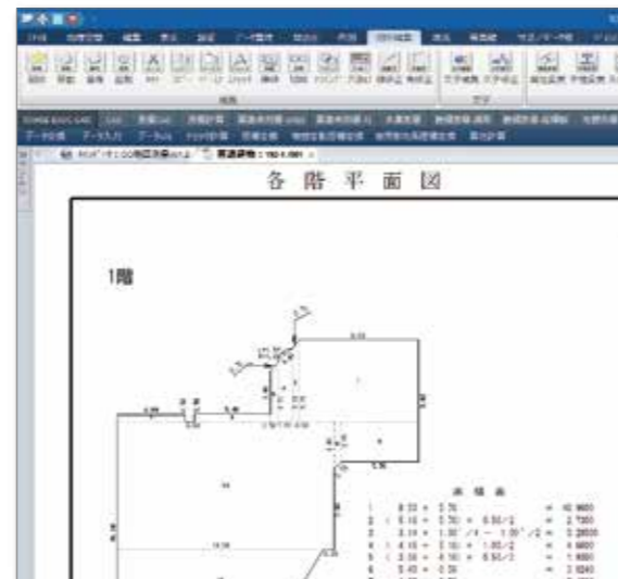
建物図面
